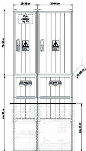
WIDOK ZESTAWU ZŁĄCZOWO - POMIAROWEGO
