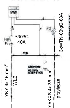
SCHEMAT STRUKTURALNY
